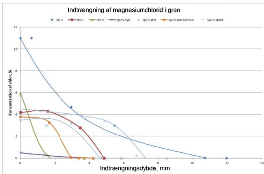
Figur 10. Indtrængningsdybde af \text{MgCl}_2 i gran efter ca. 1 år. Magnesiumkloriden trænger i første omgang kun få mm ind i træet, men kan trænge op til 10 mm ind ved længere tids påvirkning af f.eks. en
