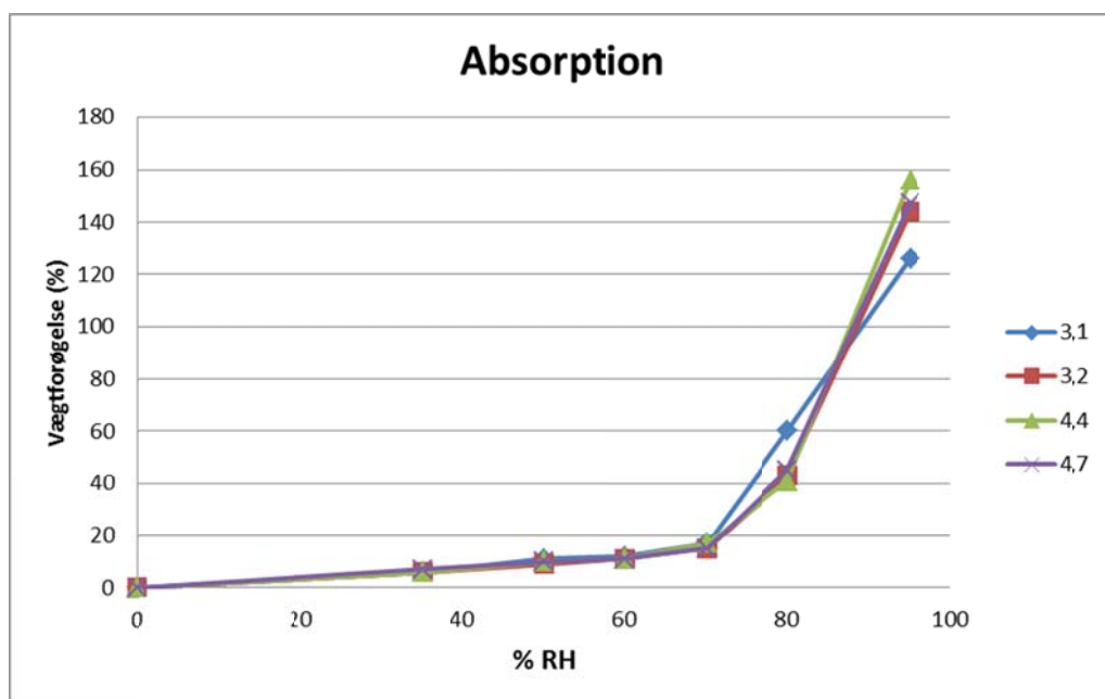
Figur 8: En foreløbig ligevægtskurve fra DTU.
